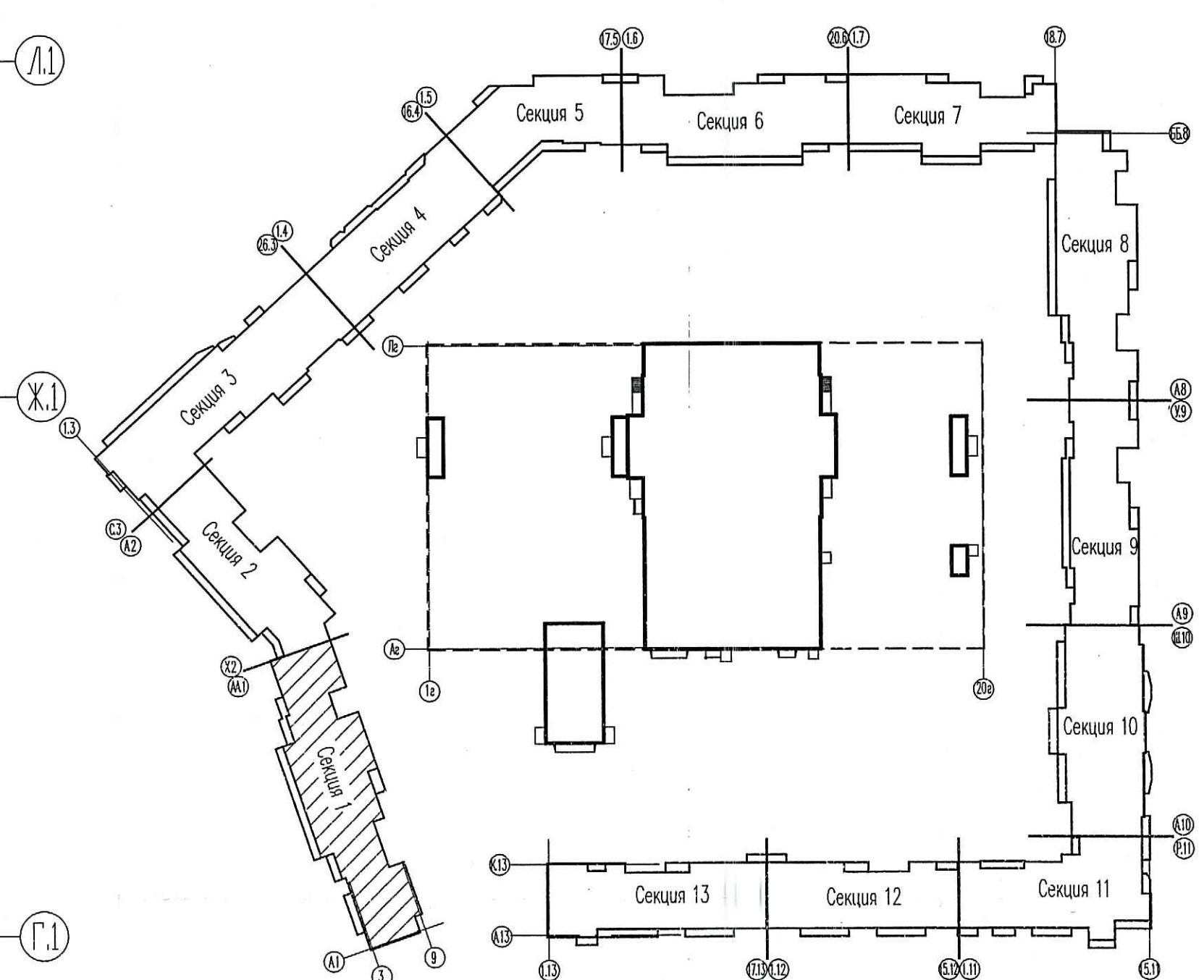
Схема расположения секции
