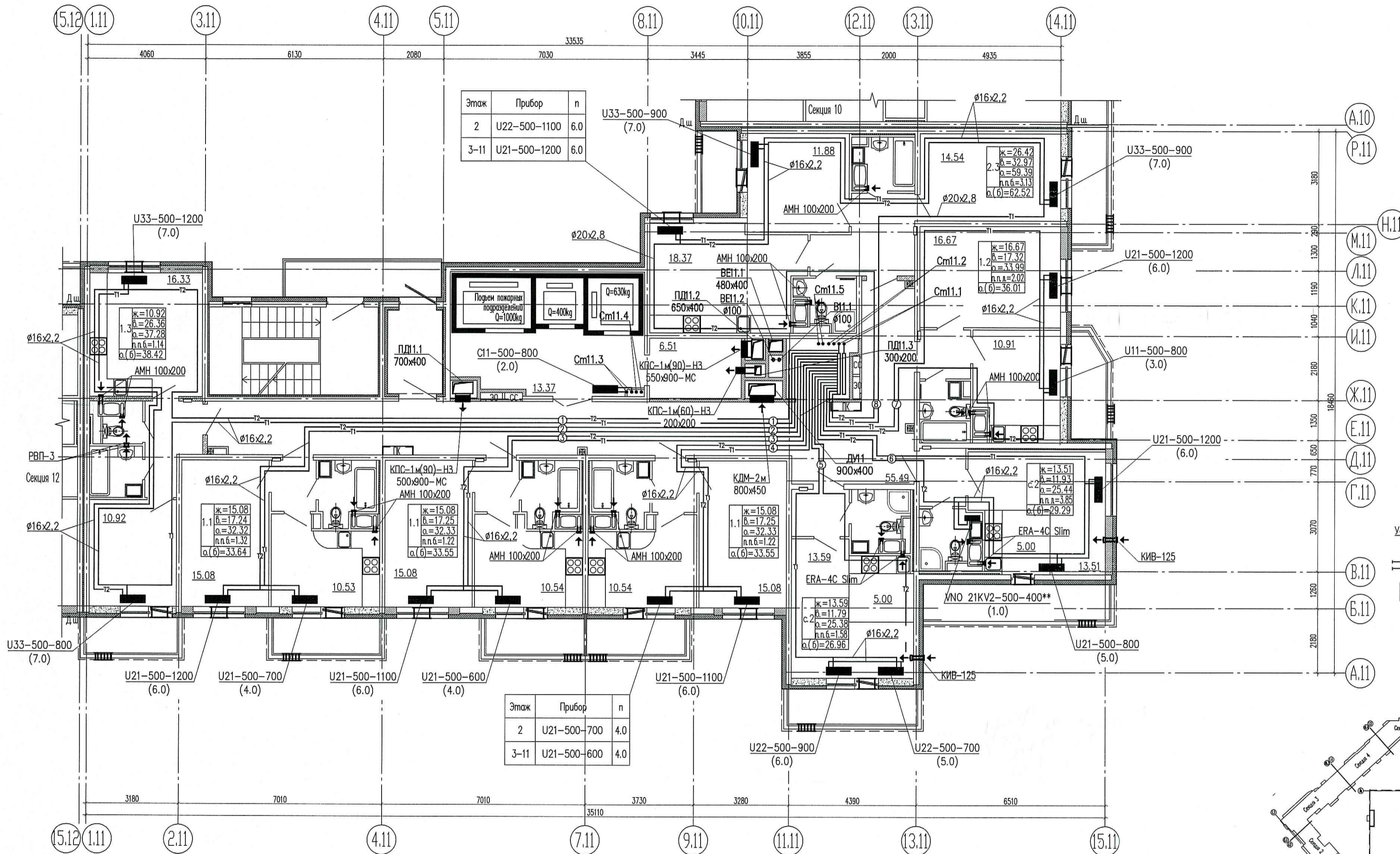
Фрагмент 1. План 11 этажа (коллектор в осях 8.11-10.11)
