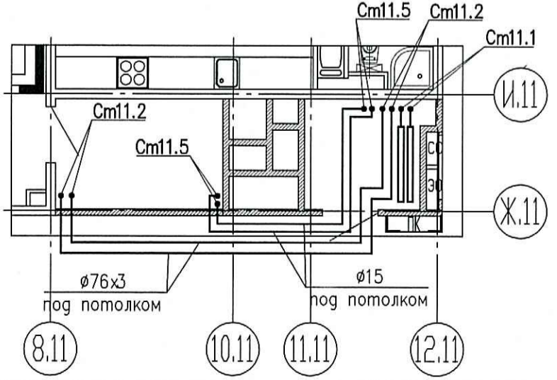
Фрагмент 1. План 11 этажа (коллектор в осях 8.11-10.11)
