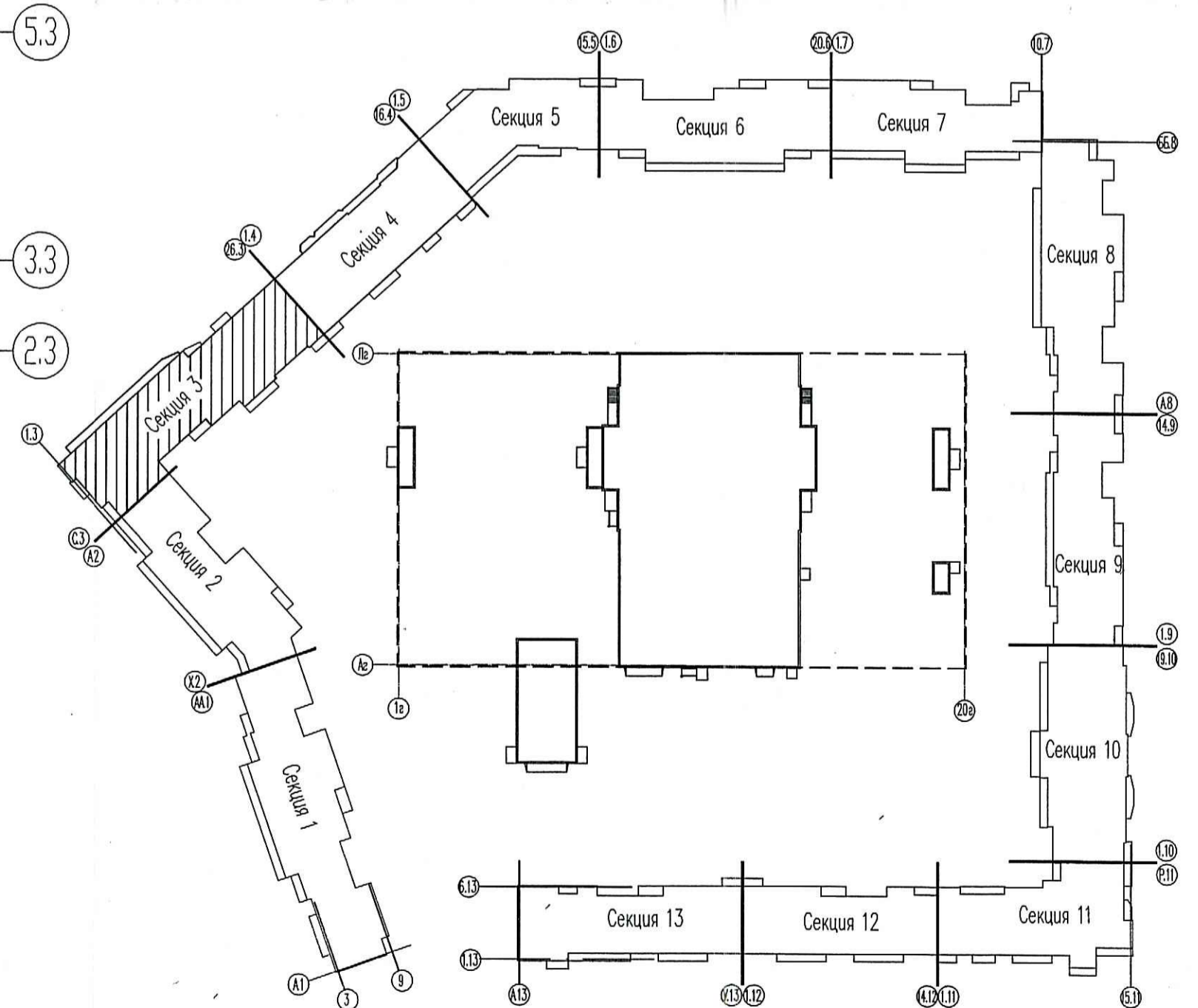
СХЕМА КОРПУСА
