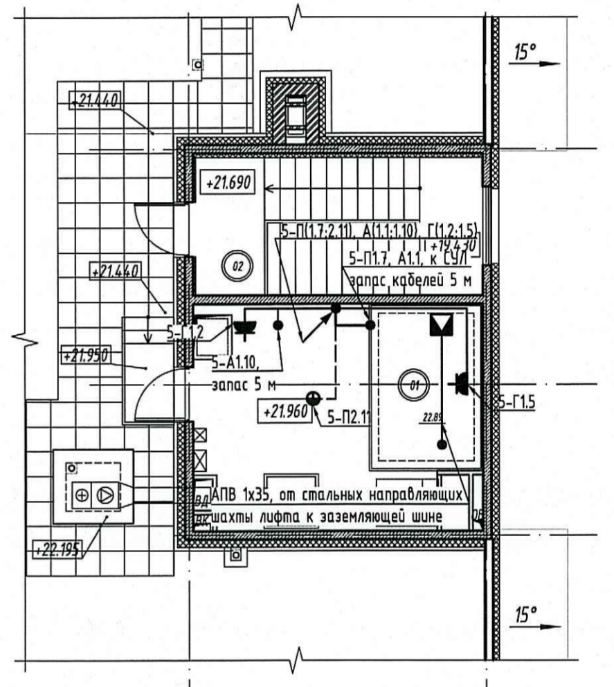
Секция 1. Машинное помещение. Выход на кровлю
