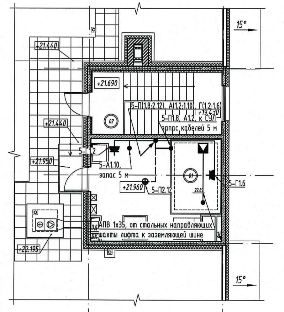
Секция 2. Машинное помещение. Выход на кровлю
